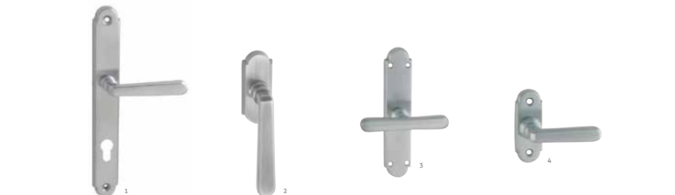
/// készleten ALT WIEN matt króm - 1. hosszúcímes 2. ablakfélkilincs 3. T-kilincs hosszú címmel 4. kis félkilincs F matt króm A réz M 1. A=112 mm B=254 mm C=33 mm 2. A=112mm B=75mm C=36mm 3. A=118 mm B= 168 mm C= 36 mm 4. A= 58 mm B= 79 mm C= 33 mm
