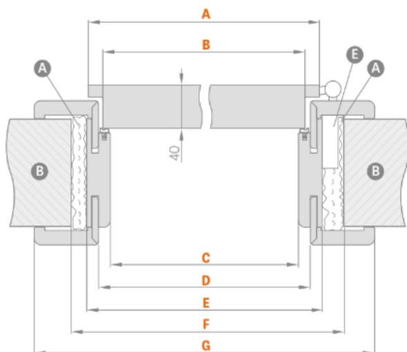
ÁLLÍTHATÓ AJTÓK ÁBRÁJA
