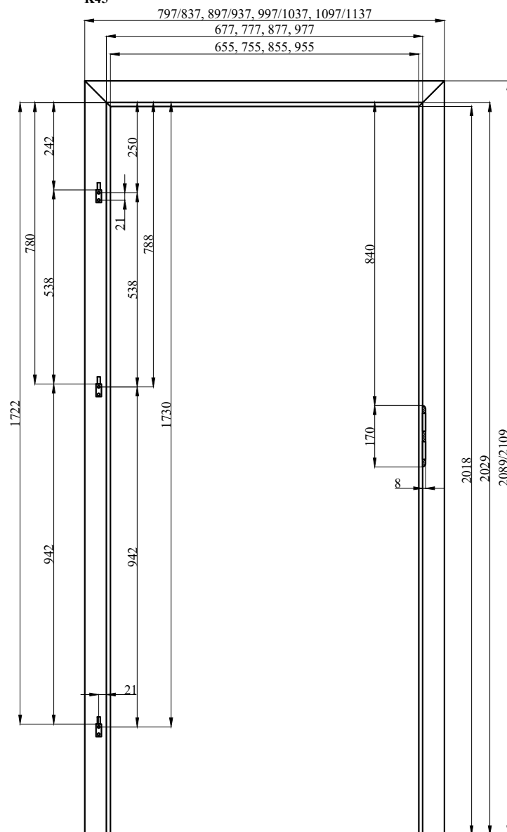
Ościeżnica regulowana przylgowa do skrzydeł "695", "795", "895", "995" K45
