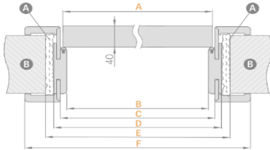
ÁLLÍTHATÓ AJTÓTOK ÁBRÁJA
