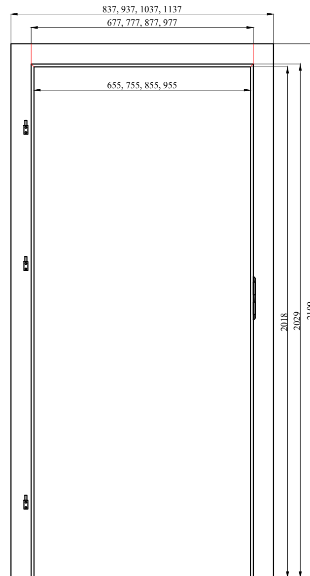
Ościeżnica regulowana przylgowa do skrzydeł "695", "795", "895", "995" K90
